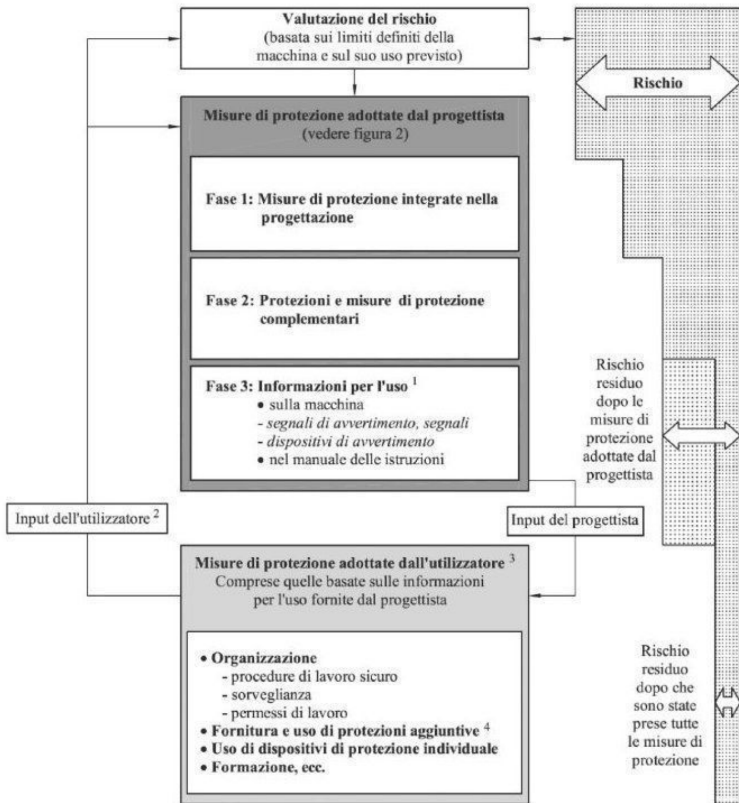
Figura 21: Processo di riduzione del rischio dal punto di vista del progettista (tratta dalla fig. 2 della norma EN ISO 12100)
