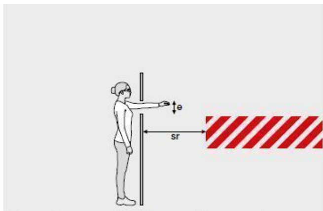
Distanze di sicurezza relative all'accesso attraverso aperture
