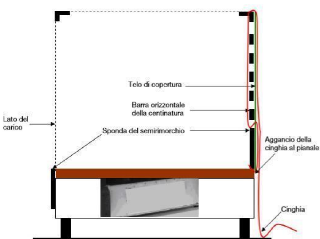
Schema 1: posizione della cinghia prima dell'inizio delle operazioni di carico ? Vista posteriore autocarro
