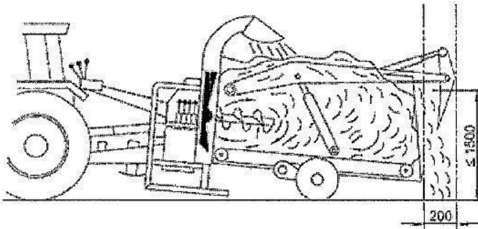
Figura 2 . Area di lavoro per la verifica della visibilità diretta per le macchine trainate. Dimensioni in mm.
