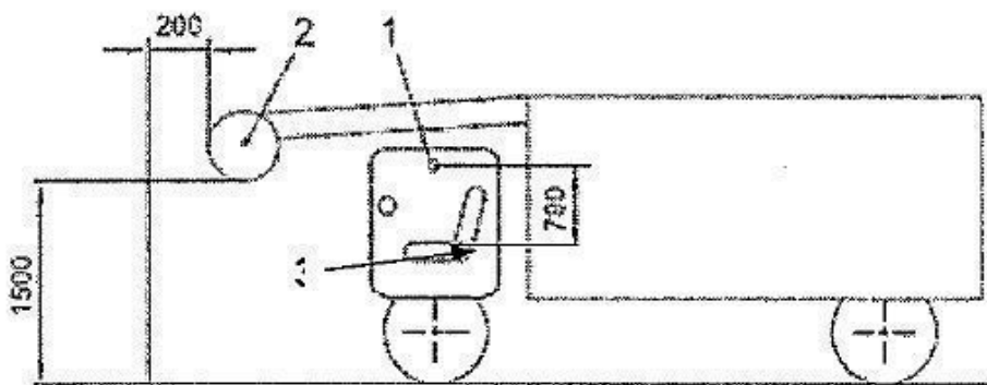
Figura 1. Area di lavoro per la verifica della visibilità diretta per le macchine semoventi. Dimensioni in mm.
