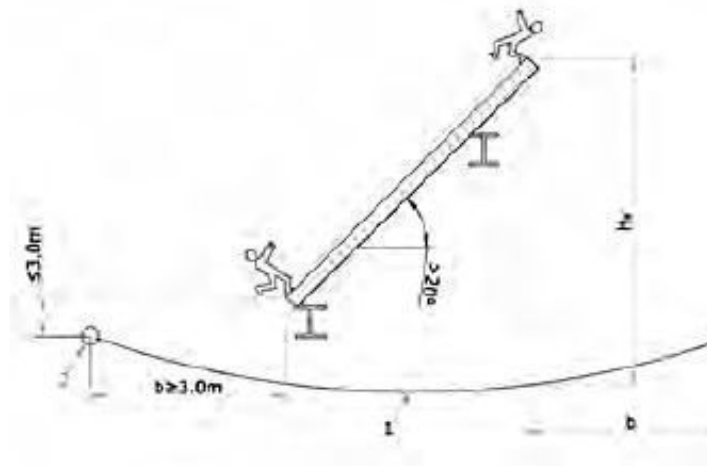
Figura 6b - Altezze di caduta ammissibili e profondità di raccolta richieste per aree di lavoro inclinate oltre i 20°
